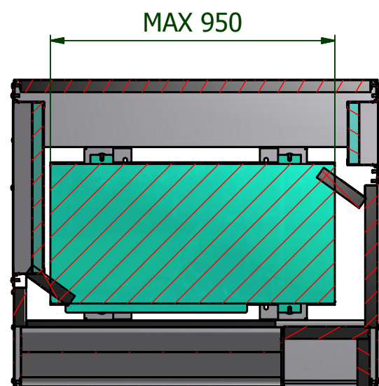
B-B ( 1 : 17.5 )
