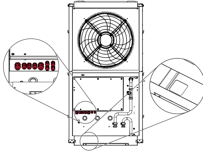
Abb. 27: Elektrische Anschlüsse in der Wärmepumpe (Symbolfoto)
