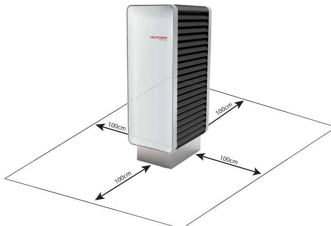
Abb. 14: Schutzbereich 1m
