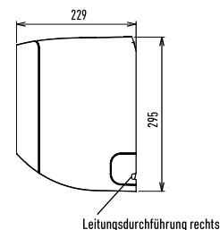
Seitenansicht
