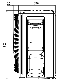
Seitenansicht
