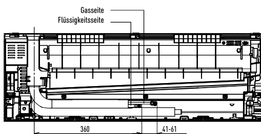
Rückansicht
