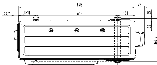
Draufsicht
